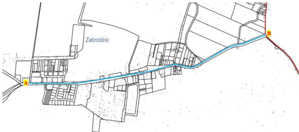
Fot. Trasa projektowanego wodociągu PEHD225 w m.Zabrodzie
