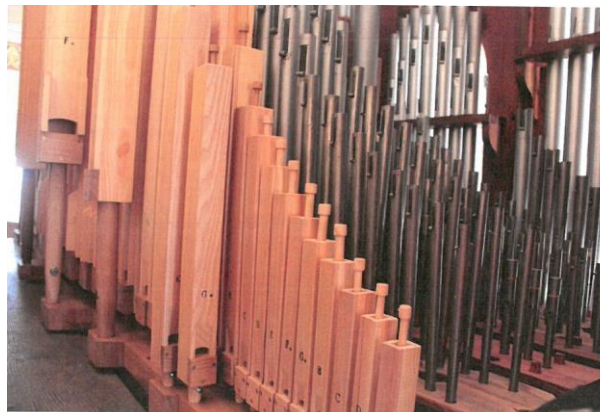
Piszczałki sekcji I i II manuatu po renowacji
