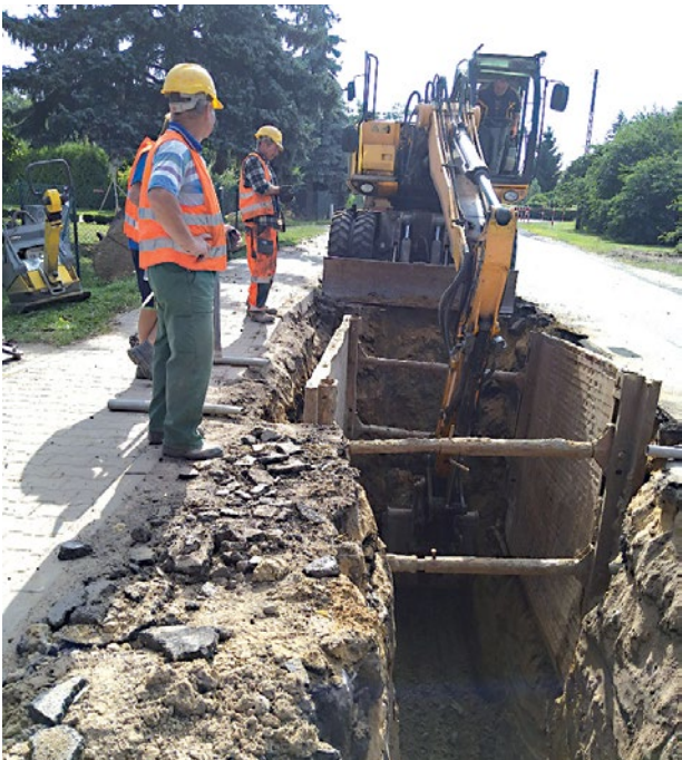
Budowa kanalizacji
